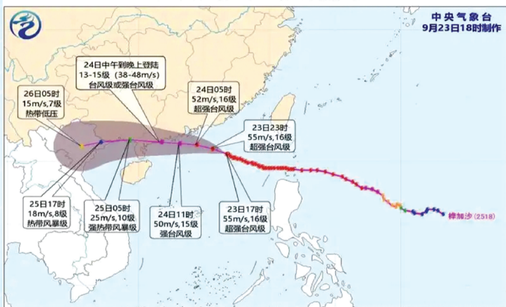
今年第18号台风“桦加沙”未来60小时路径概率预报图 2025年9月23日17时—26日05时(北京时间)
